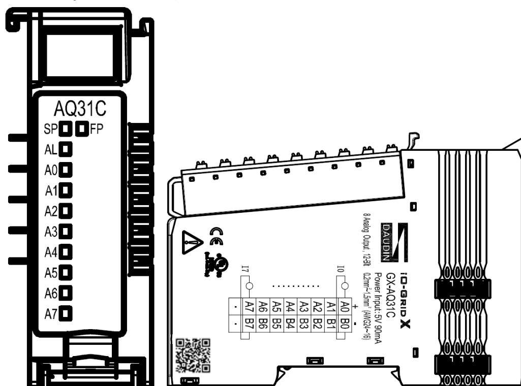
圖 4.30 GX-AQ31C 圖面
