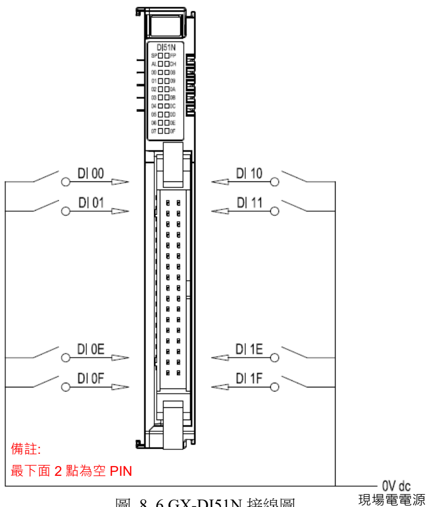
圖 8.6 GX-DI51N 接線圖
