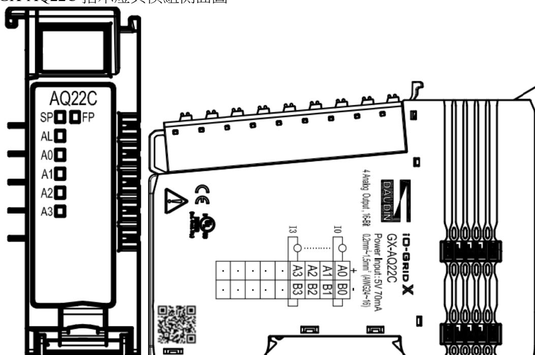
圖 4. 28 GX-AQ22C 圖面
