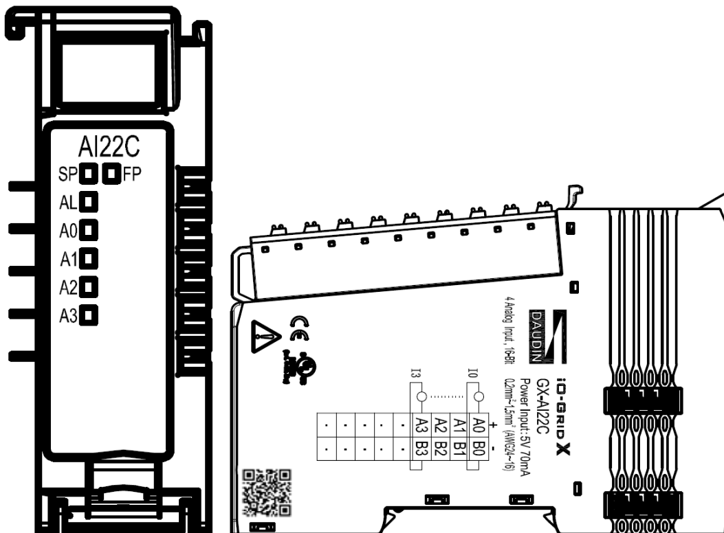
圖 4. 20 GX-AI22C 圖面
