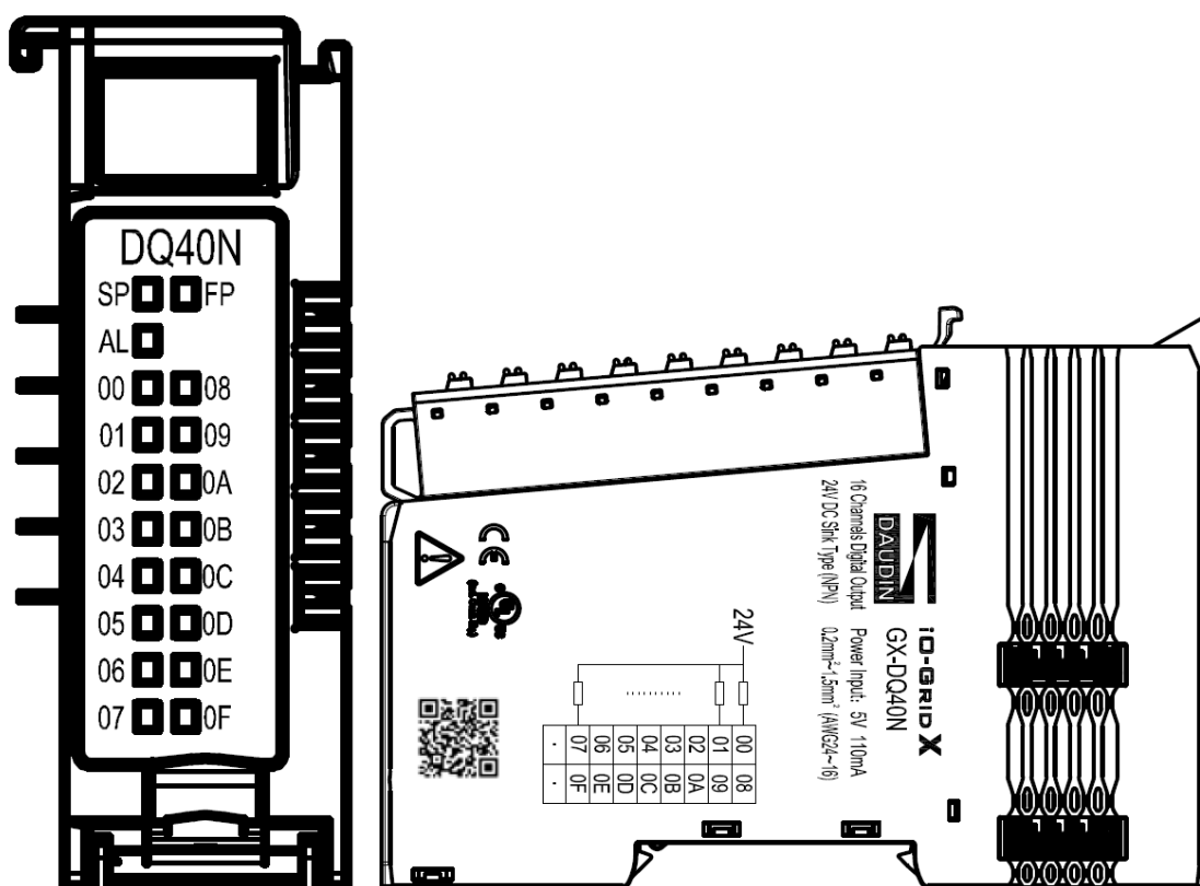
圖 4.11 GX-DQ40N 圖面
