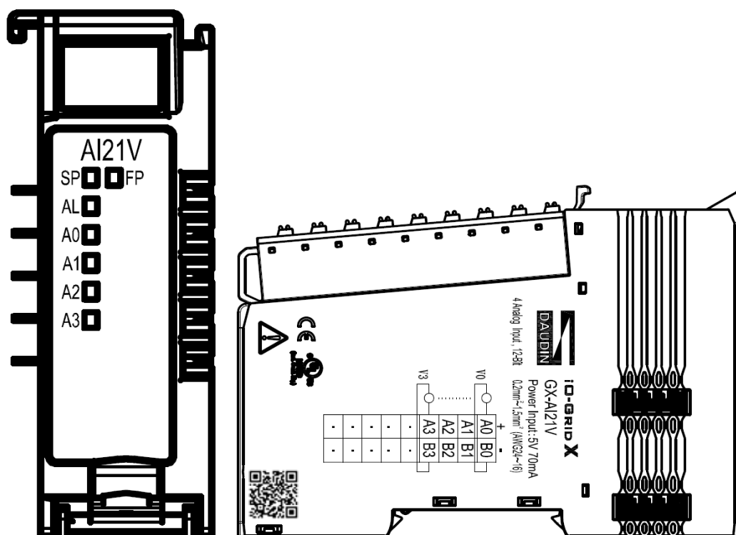
圖 4.17 GX-AI21V 圖面
