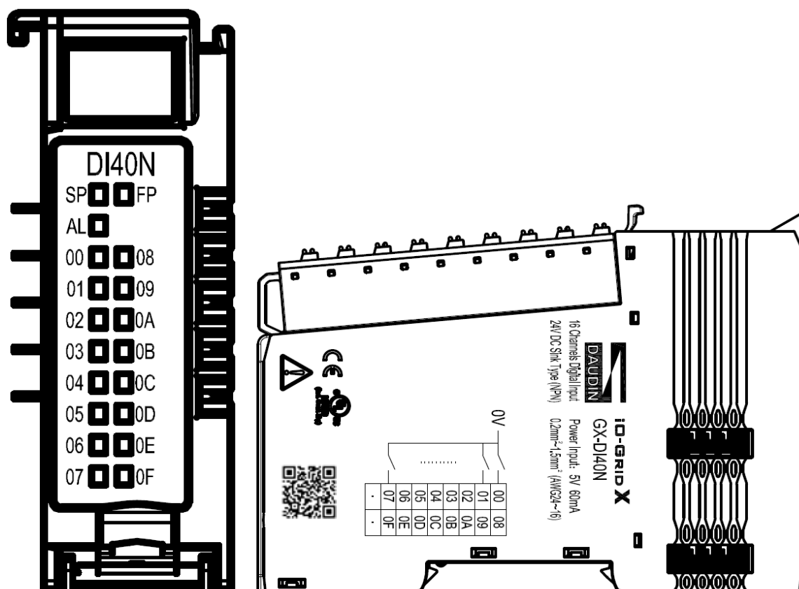
圖 4.4 GX-DI40N 圖面
