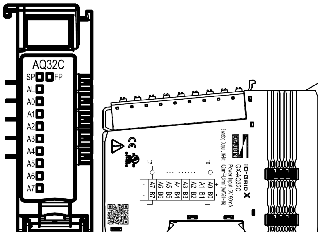
圖 4.32 GX-AQ32C 圖面
